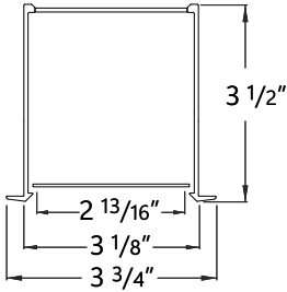
DF drywall flange shown
