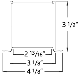
DS drywall spackle flange shown
