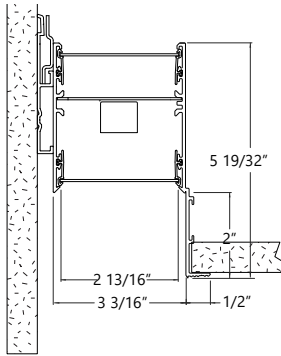
2RG 2" regressed DS Drywall spackle
