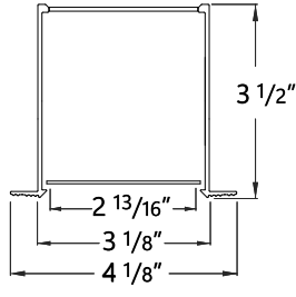
DS drywall spackle flange shown
