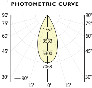
MikroLite - 4ft - 50 deg 1000 lm/ft
