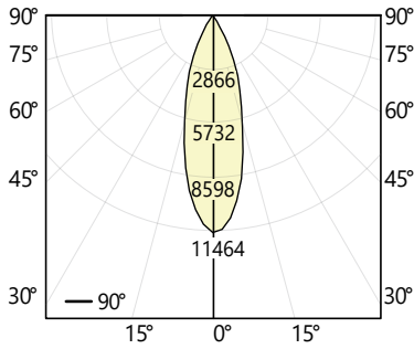
MikroLite - 4ft - 24 deg 1000 lm/ft
