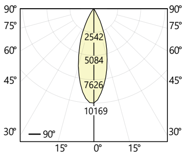
MikroLite - 4ft - 38 deg 1000 lm/ft
