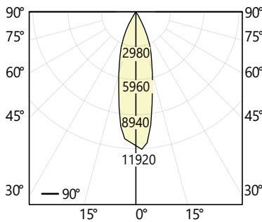
MikroLite - 4ft - 15 deg 1000 lm/ft
