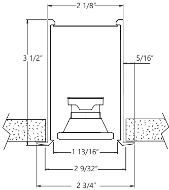
DF Drywall flange shown
