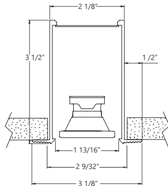
DS Drywall spackle flange shown
