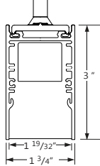
Louver shown
